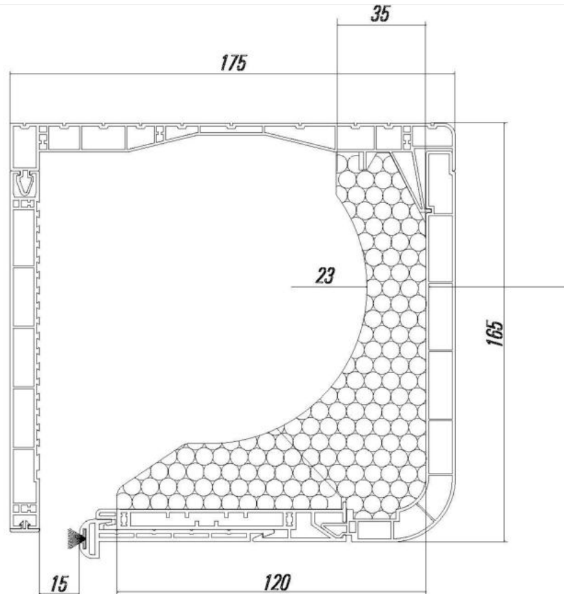
Bild 2 Schnittzeichnung
