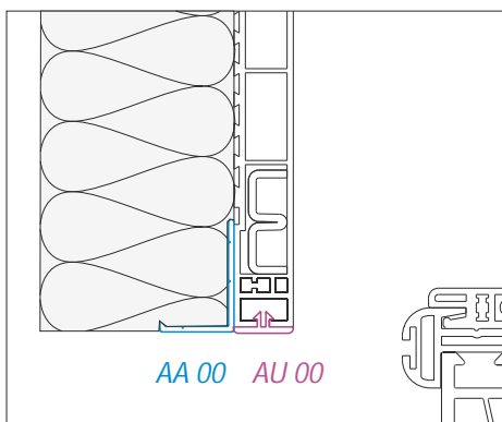
zabudowana z zewnątrz skrzynka rolety CleverBox z dotychczas stosowanym teownikiem AA 00 i załepką AU 00
