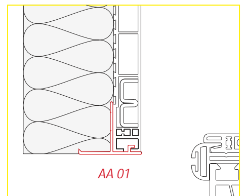
zabudowana z zewnątrz skrzynka rolety CleverBox z zastosowaniem nowego teownika AA 01
