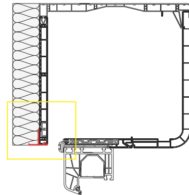
miejsce stosowania profilu teownikowego w roletcie CleverBox z pokrywą rewizyjną od tyłu
