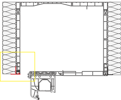
miejsce stosowania profilu teownikowego w roletcie CleverBox z pokrywą rewizyjną od dołu
