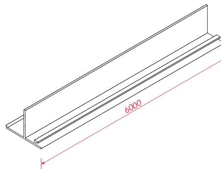
rysunek techniczny 3D prezentujący profil teownikowy
