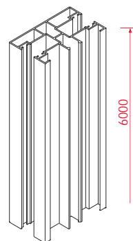
rysunek techniczny 3D prezentujący prowadnicę pancerza mini (ALU)
